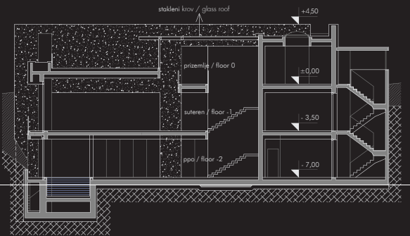
presjek / section
